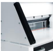
IR Light Beam เซ็นเซอร์อัจฉริยะ ที่มาแทนฝาครอบหน้าเครื่อง ทำให้ปลอดภัยในการตัดทุกครั้ง
